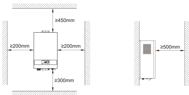
Рис. 4. Минимальные расстояния от электрического котла до поверхностей.
