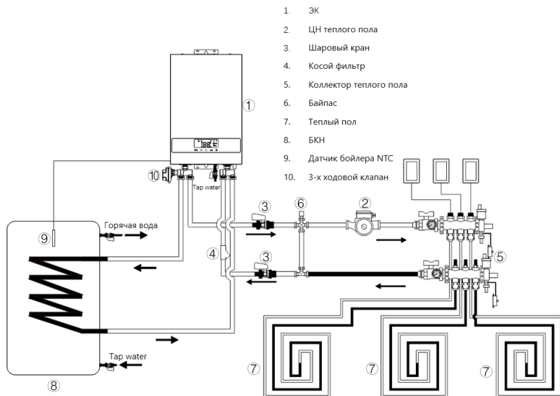
Рис. 20. Схема подключения «ЭК + БКН + Теплый пол».
