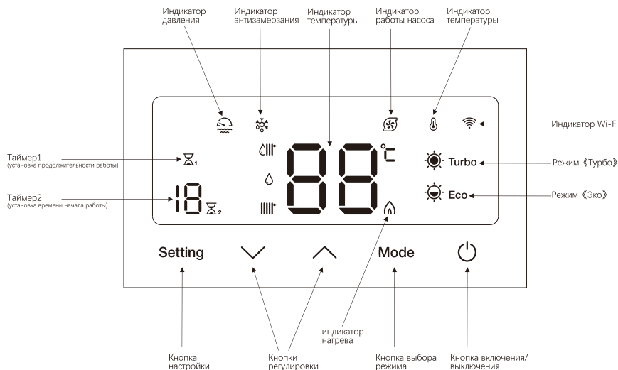
Рис. 3. Панель управления
