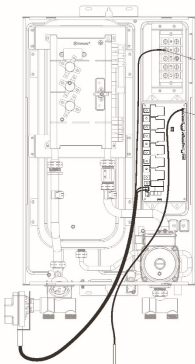
Рис. 18. Подключение датчика бойлера
