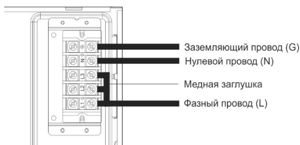
Рис 10. Однофазное подключение прибора
