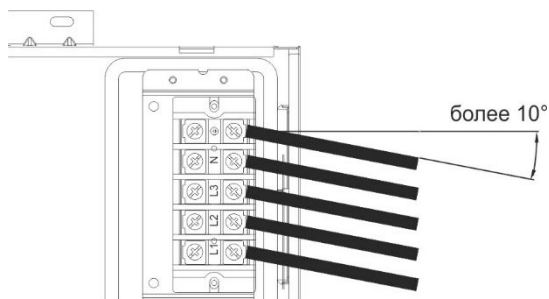
Рис. 12. Расположение сетевого кабеля
