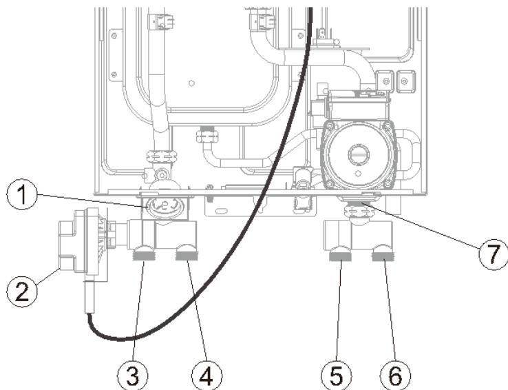
Рис.16. Присоединение трехходового клапана
