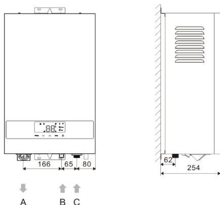
Рис. 6. Присоединительные размеры
