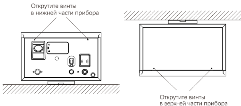
Рис. 7. Демонтаж лицевой панели
