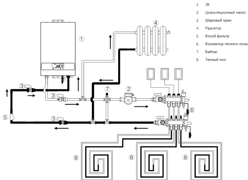
Рис. 15. Схема подключения «ЭК + Радиаторы + Теплый пол».
