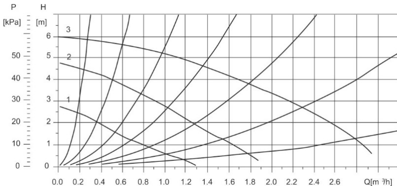
Рис. 23. Кривая характеристик давления насоса
