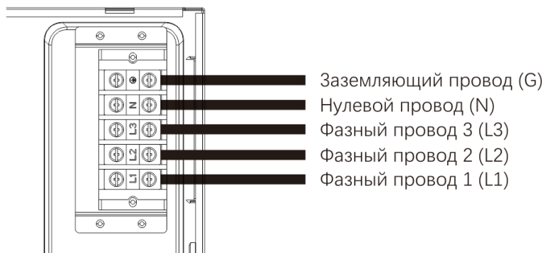
Рис 11. Трехфазное подключение прибора
