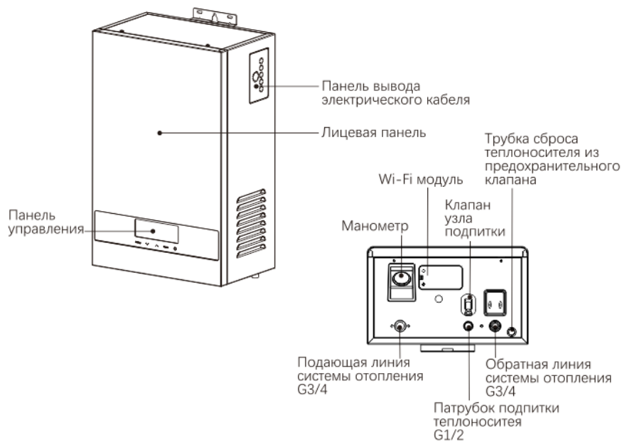
Рис. 1. Конструкция изделия
