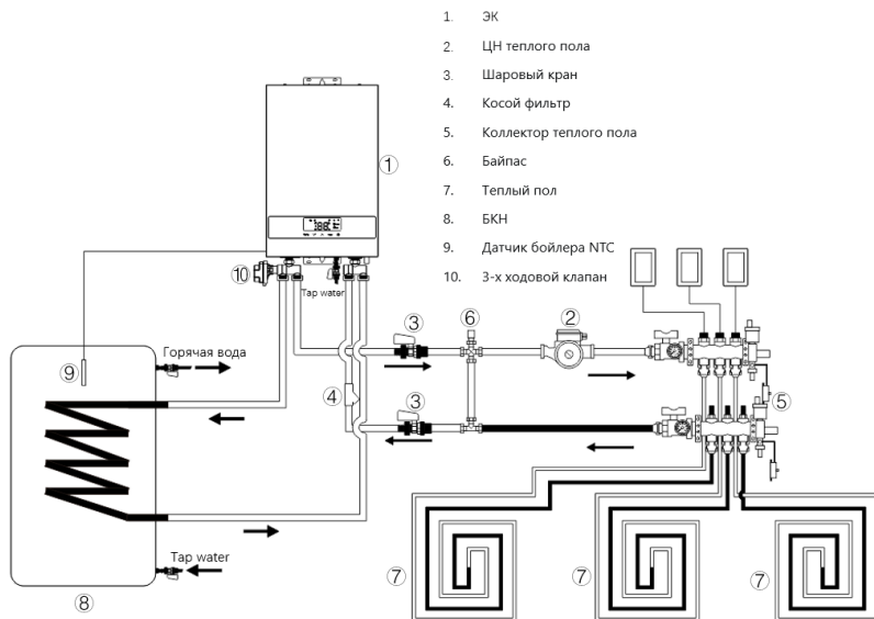
Рис. 20. Схема подключения «ЭК + БКН + Теплый пол».
