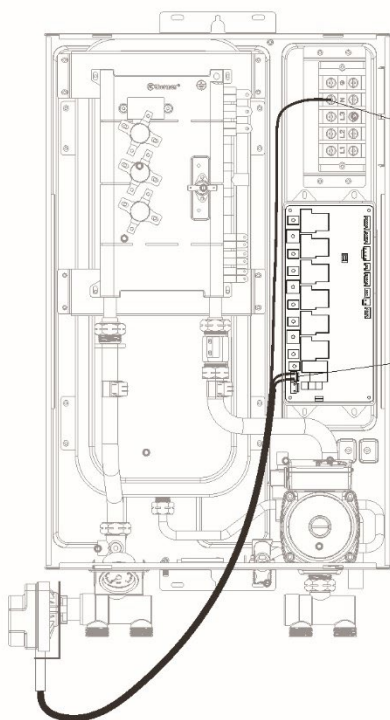
Рис. 17. Подключение трехходового клапана
