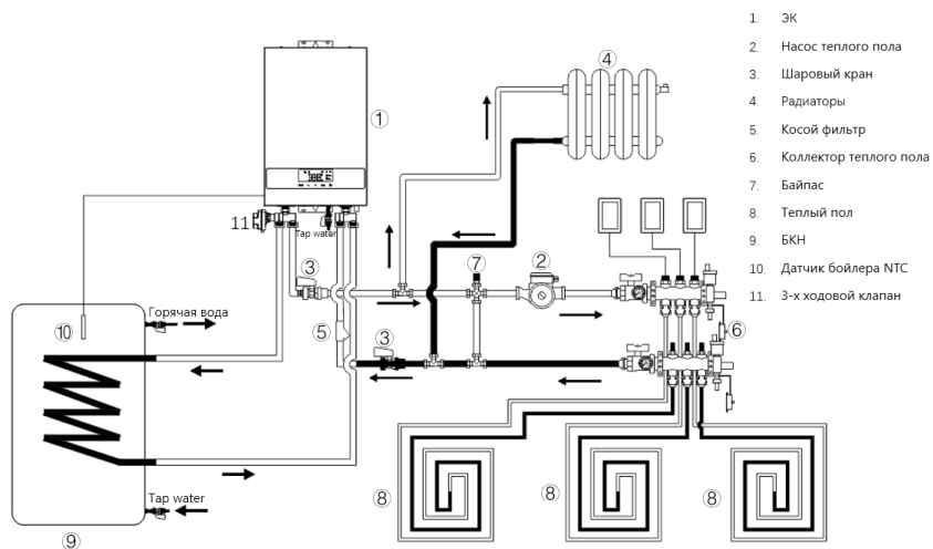
Рис. 21. Схема подключения «ЭК + БКН + Теплый пол + Радиаторы».
