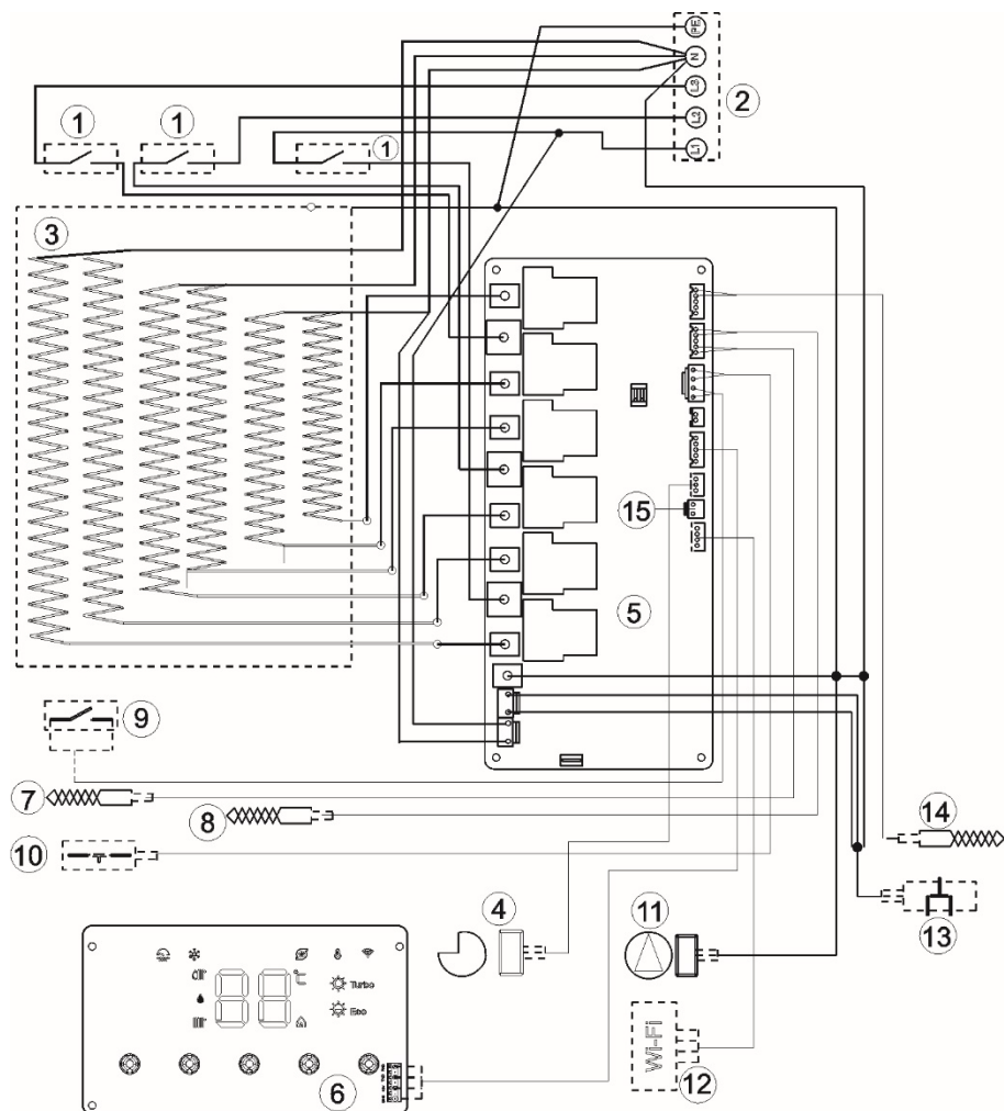
Рис. 24. Электрическая схема THERMEX Sonne 12 Wi-Fi
