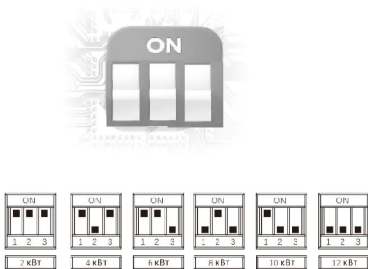
Рис. 8. Положение рычагов переключателя мощности.
