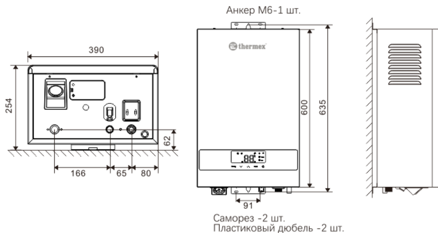
Рис. 5. Монтажные размеры
