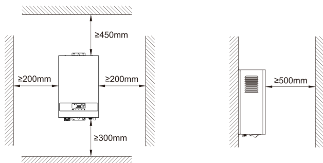
Рис. 4. Минимальные расстояния от электрического котла до поверхностей.
